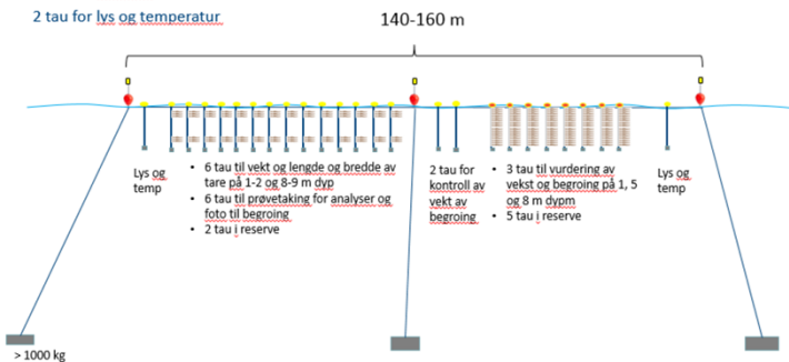
Skisse 1: Skissemessig framstilling av bøyestrekket (Utarbeidet av Macrosea), hentet fra tidligere søknad i samme prosjekt i Smalfjord (saksnr. 2016/3211).
